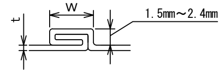
A部拡大断面図
