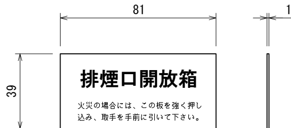
アクリル板詳細図
