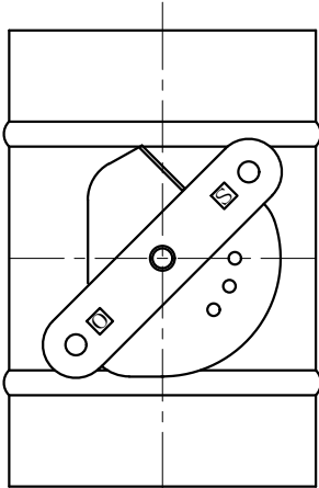
立管仕様
