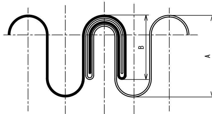
①拡大図
